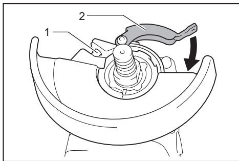
► 1. Tornillo 2. Palanca
