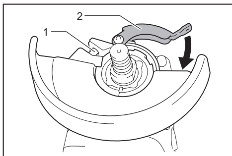
► 1. Screw 2. Lever
